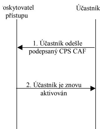
Obr. 6-4 Přejechod od provozovatele CPS k společnosti v síti CETIN
