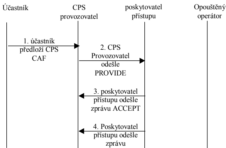
Obr. 6-6 Změna provozovatele CPS
